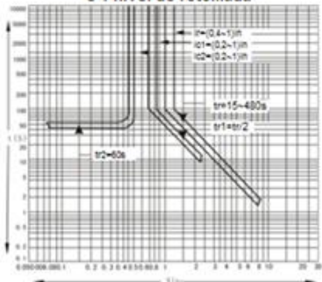
1 nível de limite de carga e 1 nível de retomada
